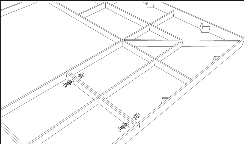
Afb. 11 Inlegframe bouten DIN933 M12 ringen DIN125 moeren DIN934 M12
