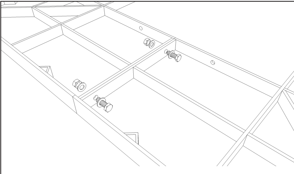
Afb. 5 Inlegframe bouten DIN933 M12 ringen DIN125 moeren DIN934 M12
