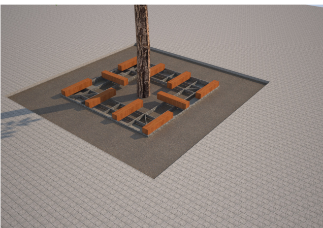
abb. 7 Provisorische Balken
