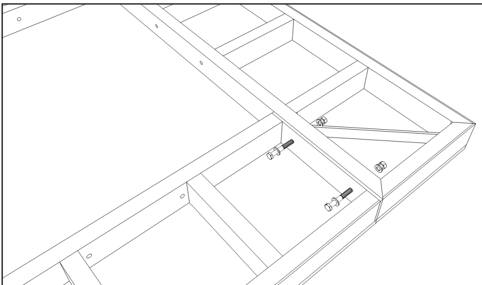
Abb. 12 Schwere Unterkonstruktion
