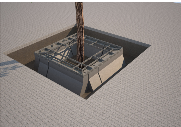
abb. 6 Unterkonstruktion
